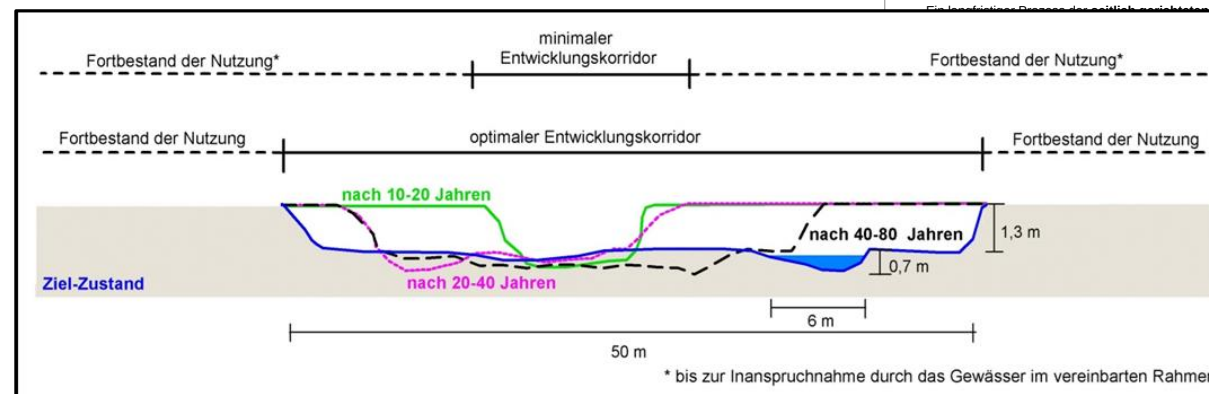
Schematische Darstellung der baulichen Entwicklung einer Sekundäraue
