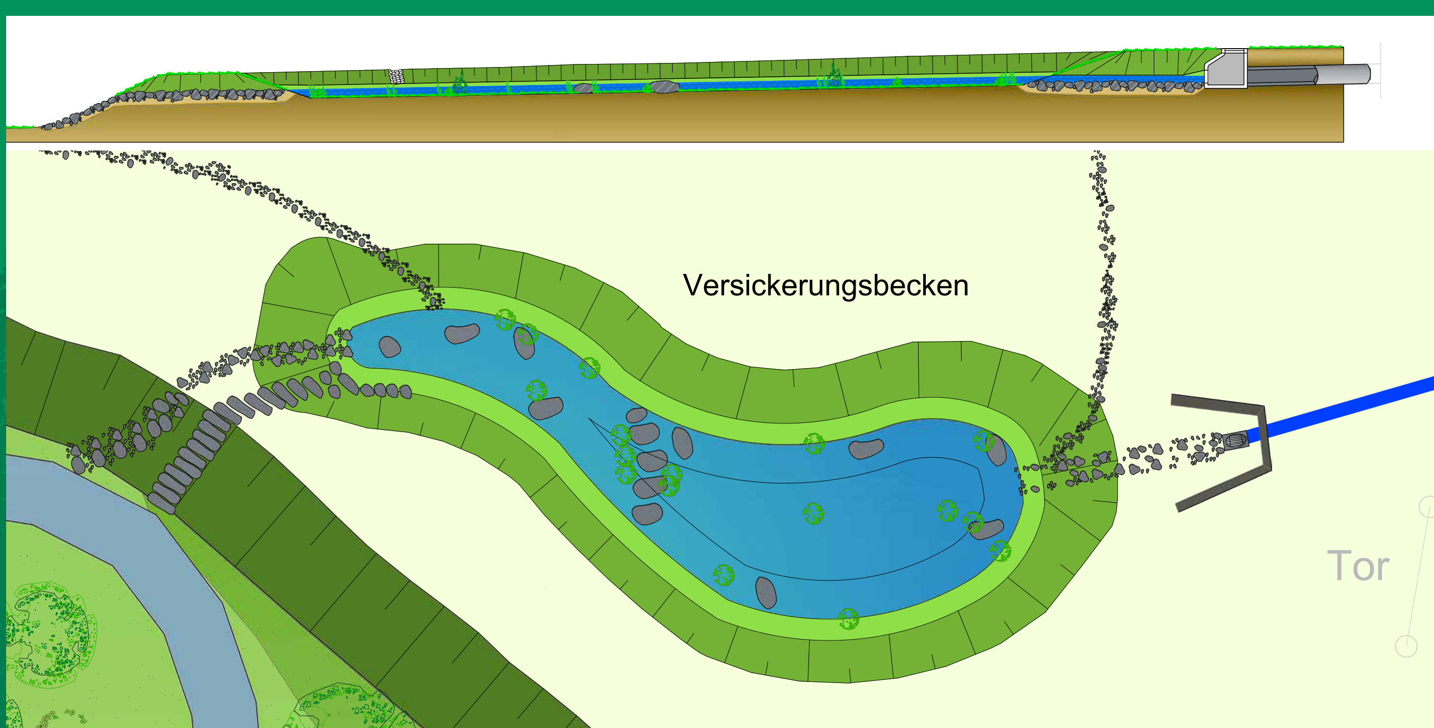
Detailskizze Versickerungsbecken
